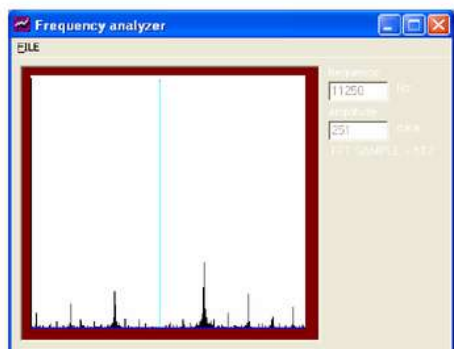
Gambar 5. Pengujian Frekuensi pada 11.250Hz
