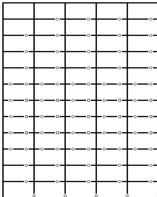
Gambar 5.29 Lokasi Terjadinya Sendi Plastis dari Hasil Analisis Pushover untuk Bangunan 12-lantai pada Portal Interior 100 Tahun
