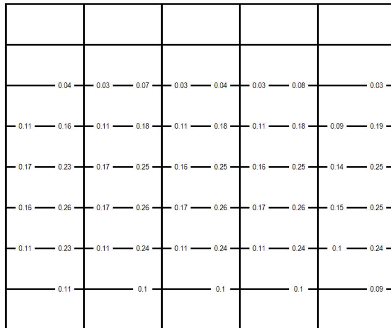
Gambar 5.17 Lokasi Terjadinya Sendi Plastis dari Hasil Analisis Time History untuk Bangunan 8-lantai pada Portal Eksterior 100 Tahun
