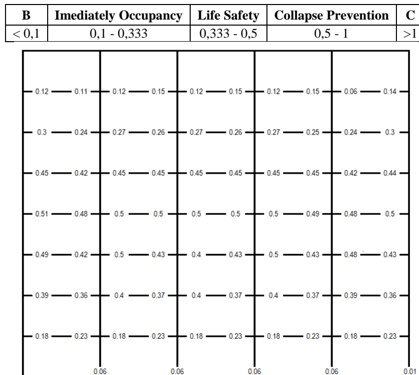
Gambar 5.23 Lokasi Terjadinya Sendi Plastis dari Hasil Analisis Time History untuk Bangunan 8-lantai pada Portal Interior 500 Tahun
