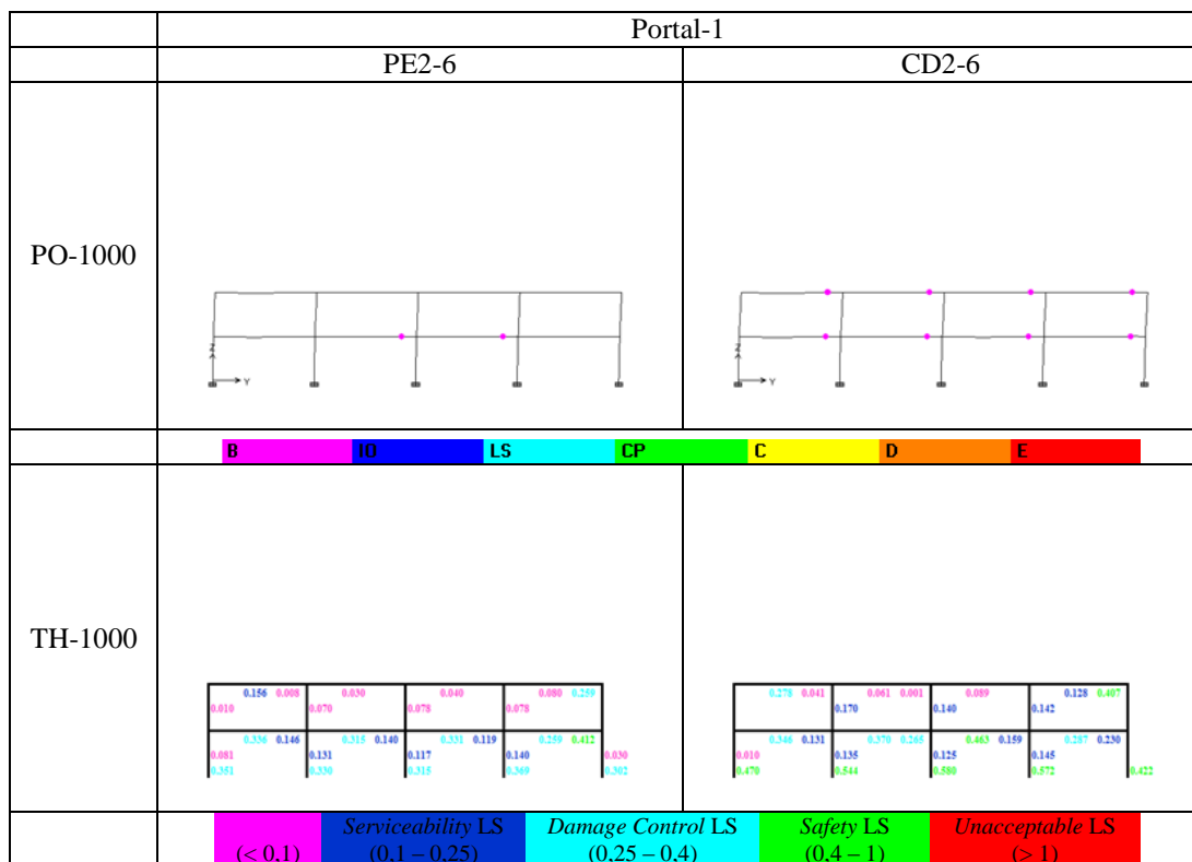
Gambar L.10 Lokasi Sendi Plastis dan Damage Index Portal 1, Gempa 1000-tahun
