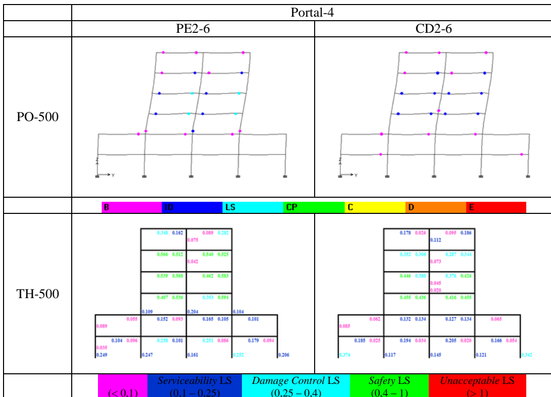
Gambar L.8 Lokasi Sendi Plastis dan Damage Index Portal 4, Gempa 500-tahun
