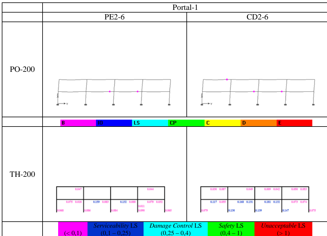
Gambar L.4 Lokasi Sendi Plastis dan Damage Index Portal 1, Gempa 200-tahun
