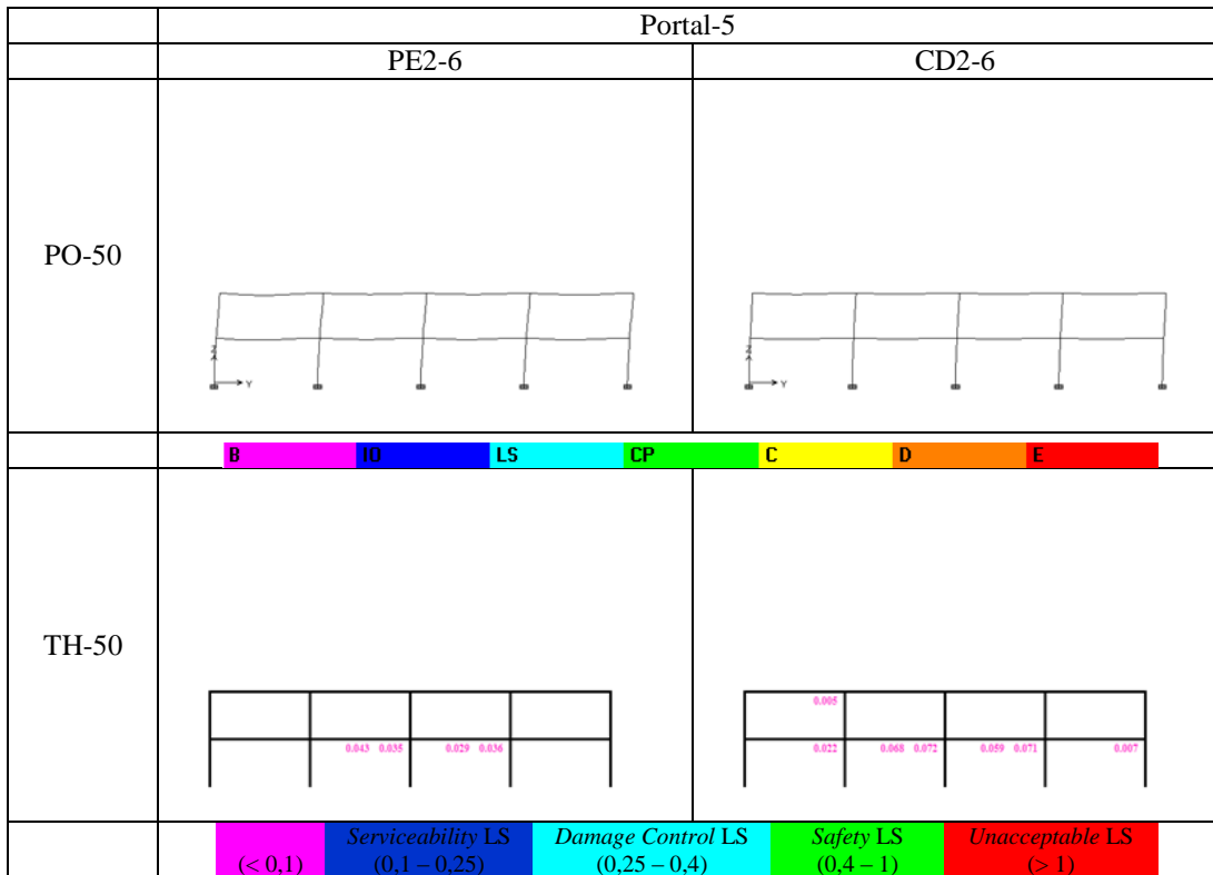
Gambar L.3 Lokasi Sendi Plastis dan Damage Index Portal 5, Gempa 50-tahun
