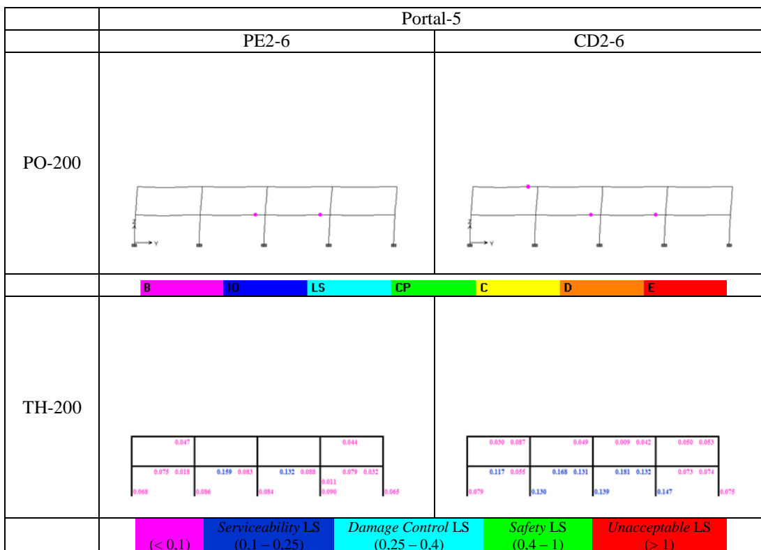
Gambar L.6 Lokasi Sendi Plastis dan Damage Index Portal 5, Gempa 200-tahun
