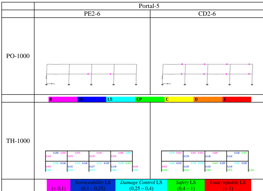
Gambar L.12 Lokasi Sendi Plastis dan Damage Index Portal 5, Gempa 1000-tahun
