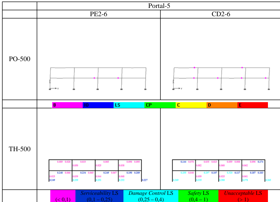
Gambar L.9 Lokasi Sendi Plastis dan Damage Index Portal 5, Gempa 500-tahun
