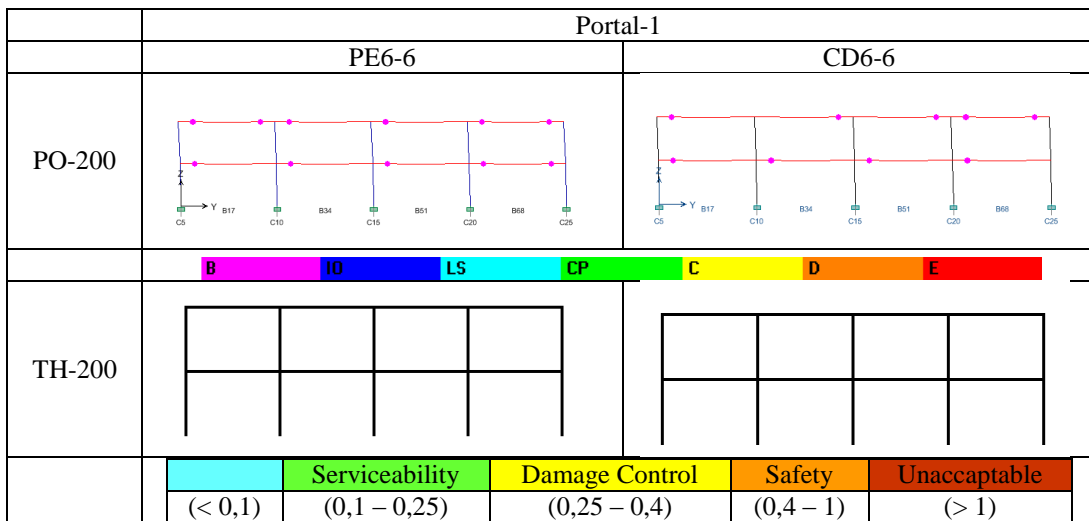
Gambar L.2 Lokasi Sendi Plastis dan Damage Index Portal 1, Gempa 200-tahun
