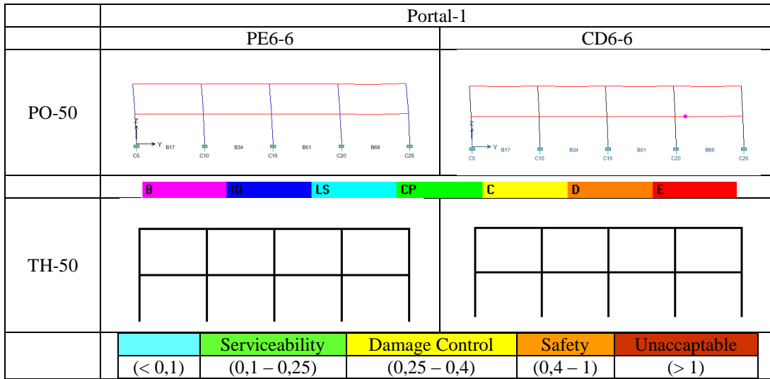
Gambar L.1 Lokasi Sendi Plastis dan Damage Index Portal 1, Gempa 50-tahun
