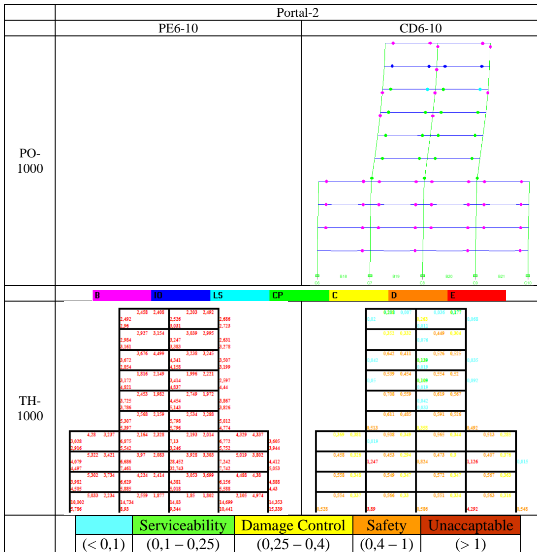
Gambar 5.20 Lokasi Sendi Plastik dan Damage Index Portal 2, Bangunan 10-lantai, Gempa 1000-tahun
