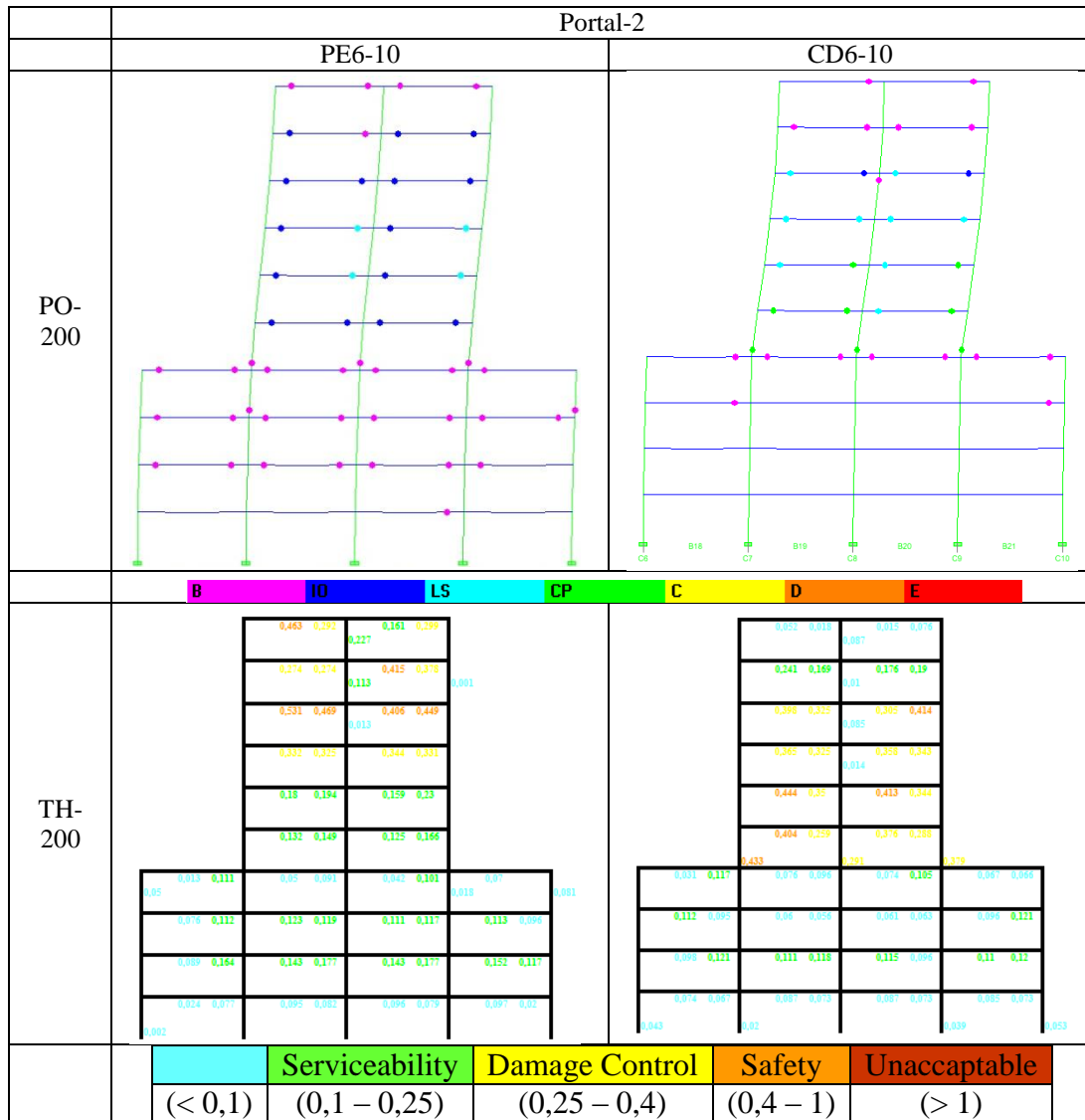
Gambar 5.16 Lokasi Sendi Plastik dan Damage Index Portal 2, Bangunan 10-lantai, Gempa 200-tahun
