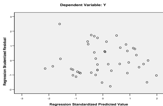
Gambar 3.2 Uji Heteroskedastisitas Dengan Scatter Plot
