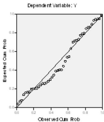
Gambar 3.1 Uji Normalitas Dengan Normal Probability Plot
