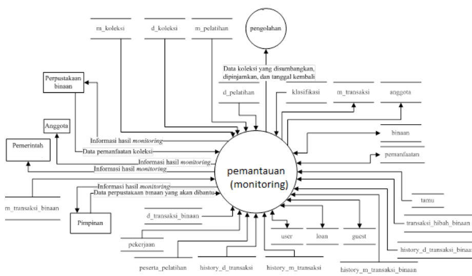
Gambar 1. DFD proses pemantauan pemanfaatan koleksi
