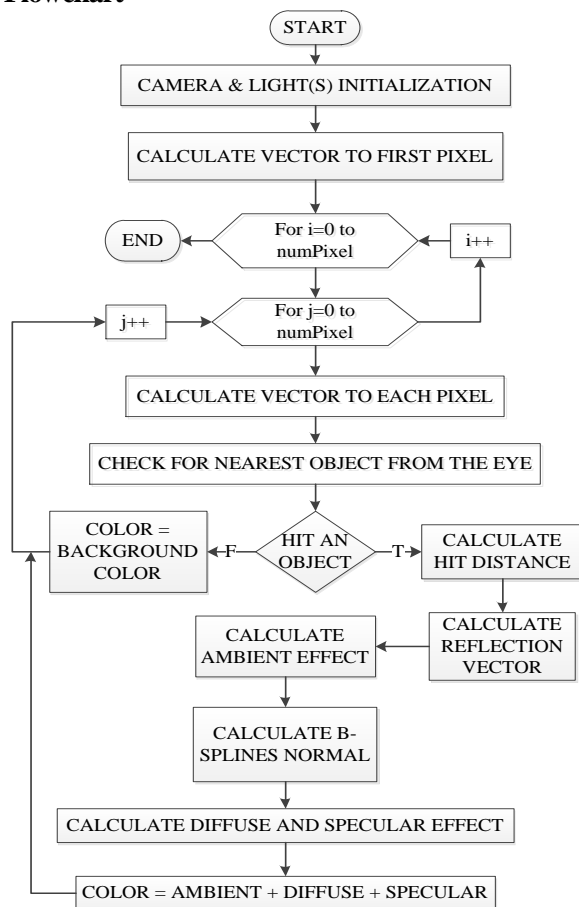
Gambar 2. Flowchart Ray tracing dengan perhitungan Normal Spline
