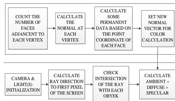
Gambar 1. Arsitektur sistem
