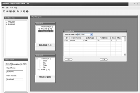
Gambar 4. Aplikasi SOM
