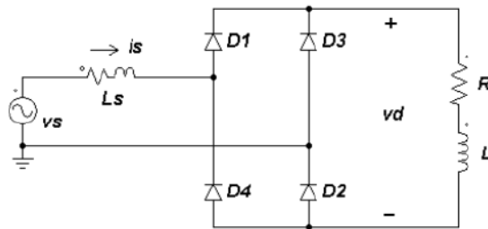
Gambar 1. Rectifier dengan induktansi sumber L_s
