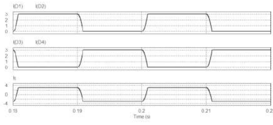
Gambar 3 Arus dioda i(D) dan arus sumber i_s
