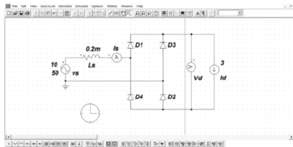
Gambar 2. PSIM: Rectifier dengan induktansi sumber L_s
