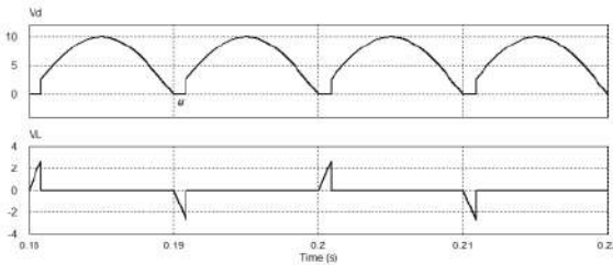
Gambar 4. Tegangan v_d dan tegangan pada L_s ( v_L )
