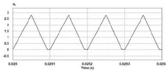
Gambar 9. L_1 < L_{(min)} , arus induktor I_L pada kondisi discontinuous conduction
