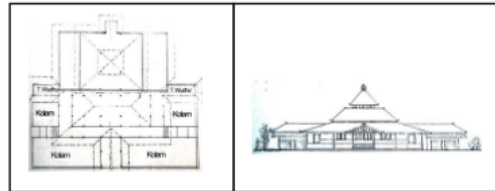
Gambar 3. Denah & Tampak Muka Masjid Ploso Kuning (Sumber: Haryadi, Jefry, 2002)
