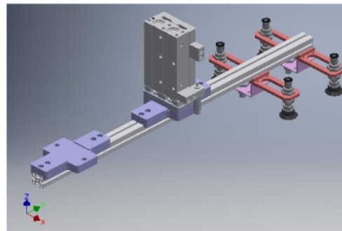
Gambar 6. Sketsa getaran arm sepanjang sumbu X
