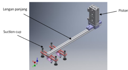
Gambar 3. Tampak isometri rencana modifikasi robotic arm
