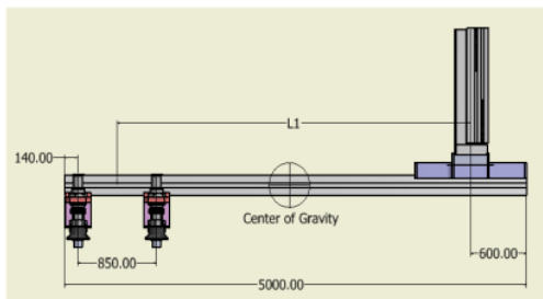
Gambar 4. Dimensi lengan sebelum modifikasi
