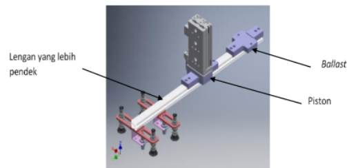
Gambar 2. Tampak isometri skets robotic arm sebelum modifikasi
