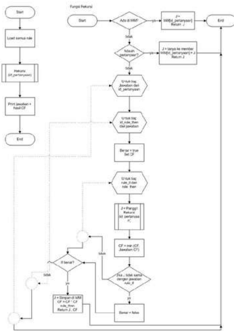
Gambar 4. Flowchart Sistem Pakar
