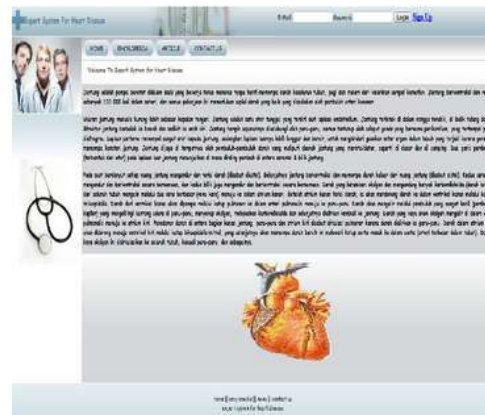
Gambar 5. Halaman Utama
