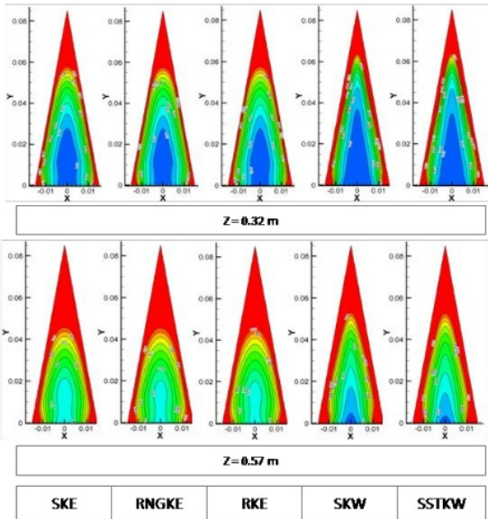
Gambar 5. Kontur temperatur pada saluran berpenampang segitiga.
