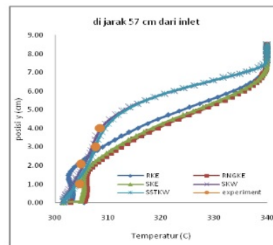
Gambar 6. Grafik distribusi temperatur di centerline .
