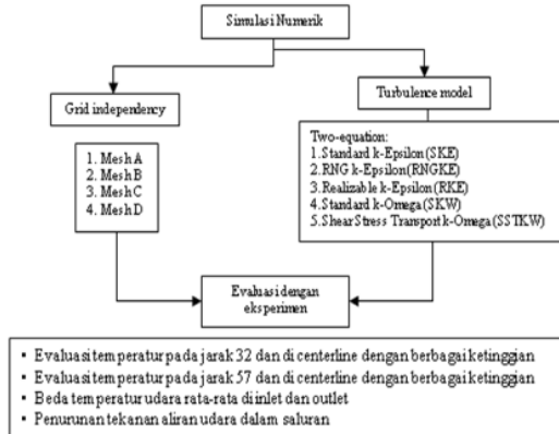
Gambar 3. Metodologi simulasi numerik penelitian ini.
