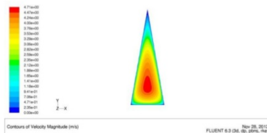
Gambar 7. Distribusi kecepatan pada jarak 0.57 m dari masukan pada centerline
