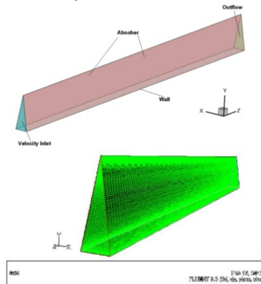
Gambar 2. Domain dan rancangan mesh yang digunakan dalam simulasi numerik.
