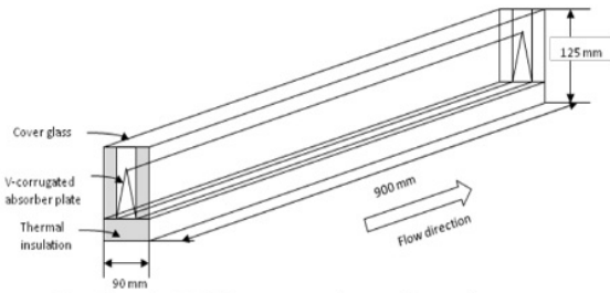
Gambar 1. (a) Skema peralatan eksperimen.
