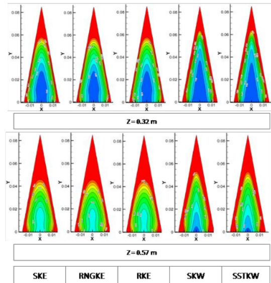
Gambar 5. Kontur temperatur pada saluran berpenampang segitiga.
