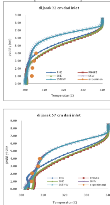
Gambar 6. Grafik distribusi temperatur di centerline .
