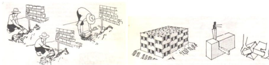
Gb. 3. Pemilihan dan Penerapan batu batako untuk dinding rumah tinggal
