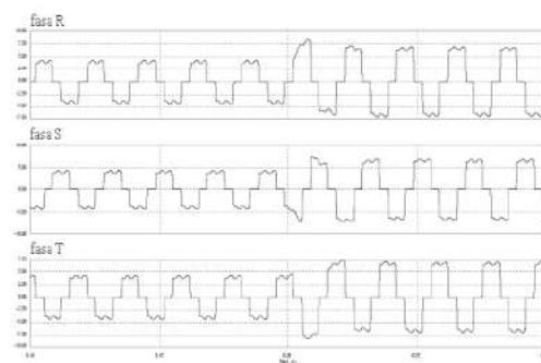
Gambar 10. Arus beban 3 fasa
