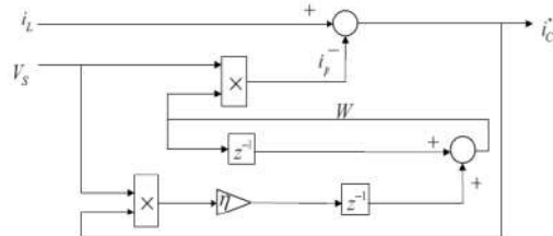
Gambar 4. Rangkaian Kompensasi i_c^*(t)
