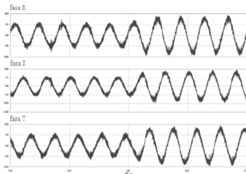
Gambar 12. Arus Sumber Setelah Kompensasi
