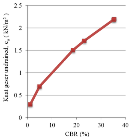
Gambar 4. Korelasi CBR dan nilai c_u
