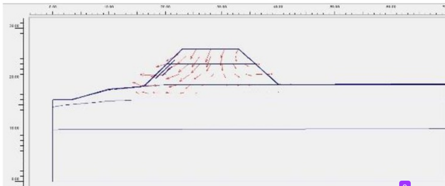
Gambar 14. Pola kelongsoran dengan kuat geser tanah timbunan rendah (kondisi MAT.3)
