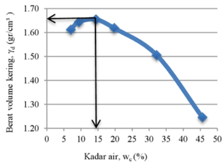
Gambar 2. Hubungan kadar air dengan berat volume kering
