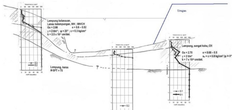
Gambar 1. Penampang waduk
