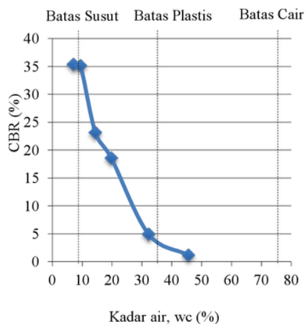
Gambar 3. Hubungan antara CBR dan kadar air
