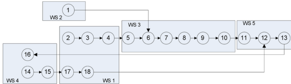
Gambar 4. Keseimbangan lintasan untuk U-Line
