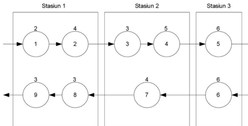
Gambar 2. Keseimbangan lintasan U-line (Gokcen, 2004)
