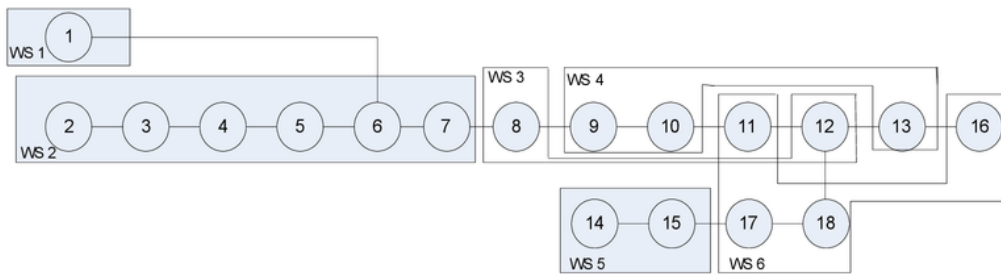
Gambar 3. Keseimbangan lintasan untuk straight line
