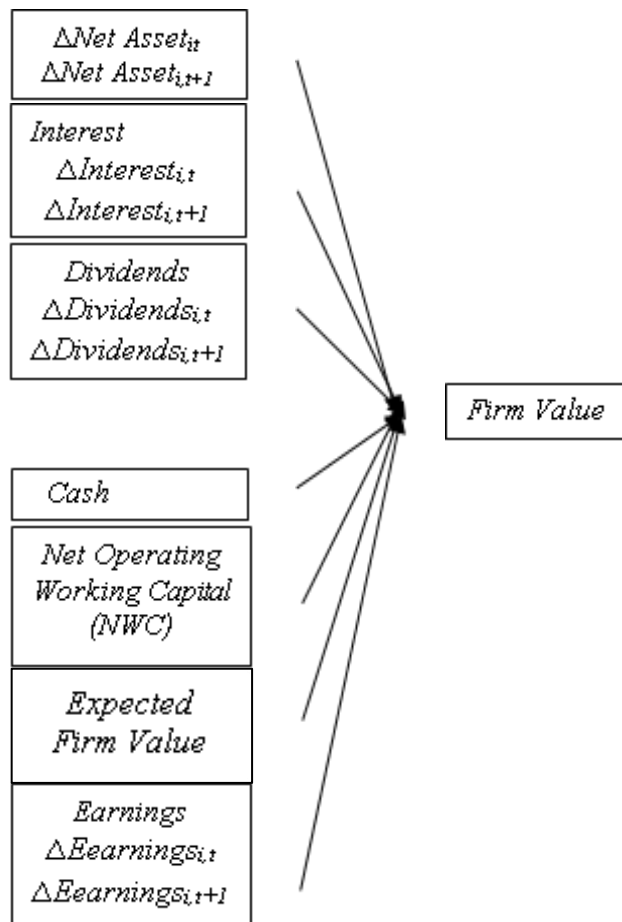
Gambar 1. Kerangka Berpikir
