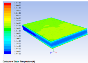
Gambar 7. Distribusi temperatur pada kolektor datar
