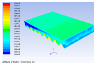
Gambar 8. Distribusi temperatur pada kolektor gelombang
