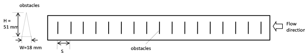
b. Gambar pandangan atas
