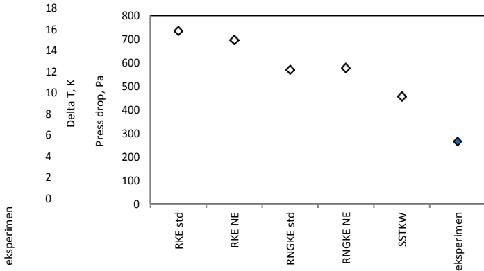
b. Penurunan tekanan aliran udara
