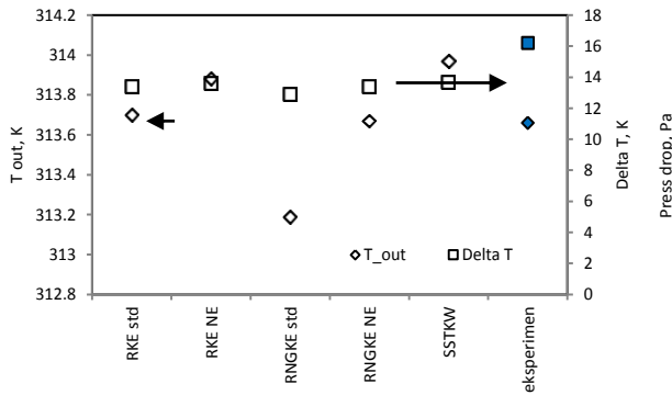
a. Temperatur ke luar dan kenaikan temperatur
