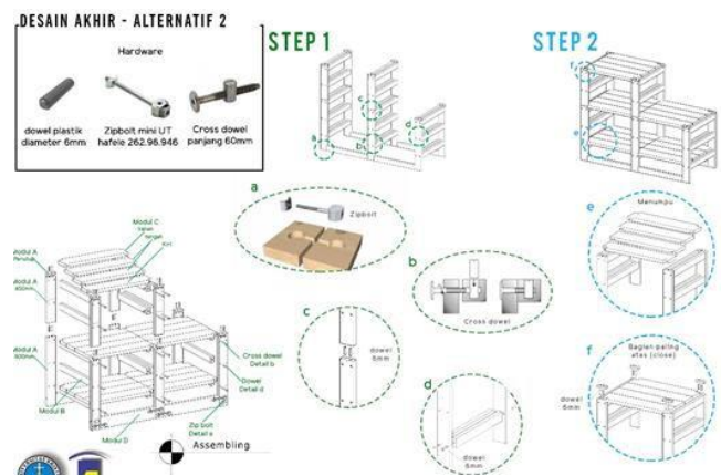
Gambar.14. Assembling dan instruksi pemasangan
