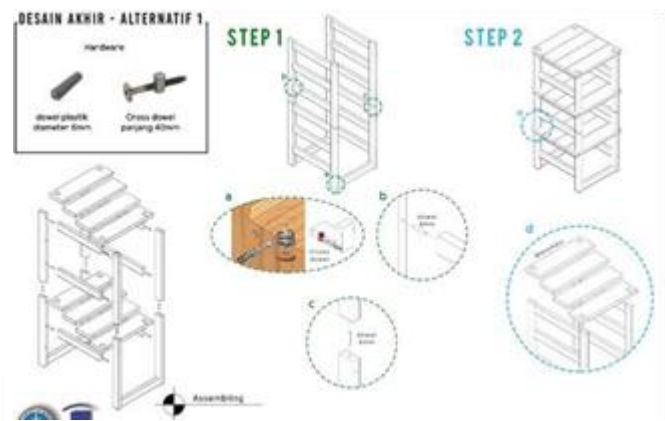
Gambar. 8. Assembling dan instruksi pemasangan
