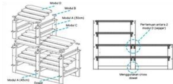
Gambar.11. Detail konstruksi transformasi desain alternatif 2
