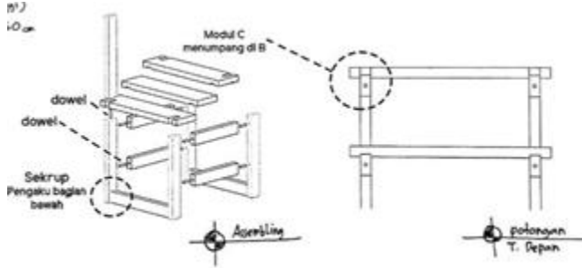
Gambar. 5. Detail konstruksi transformasi desain alternatif 1
