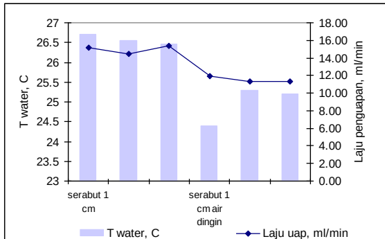
Gambar 9. Pengaruh temperatur air terhadap laju penguapan air dalam air cooler
