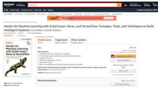
Fig. 2. Deep web.
