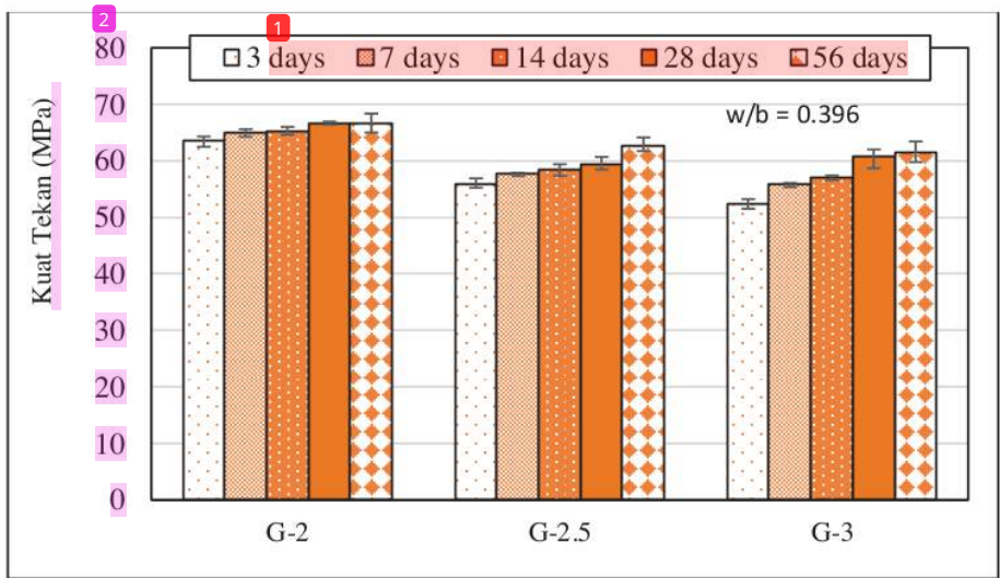
Gambar 8.3. Kuat tekan mortar geopolimer.
