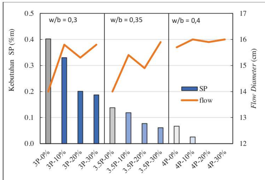
Gambar 5.1. Kebutuhan superplasticizer pada mortar pozzolan
