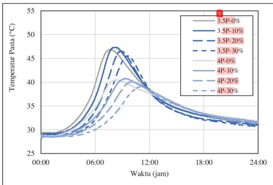
Gambar 5.3. Evolusi suhu pasta dengan variasi w/b
