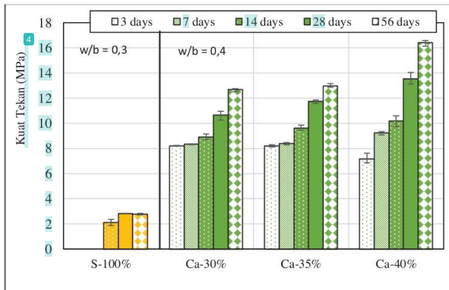
Gambar 7.4. Kuat tekan mortar Fa-Ca
