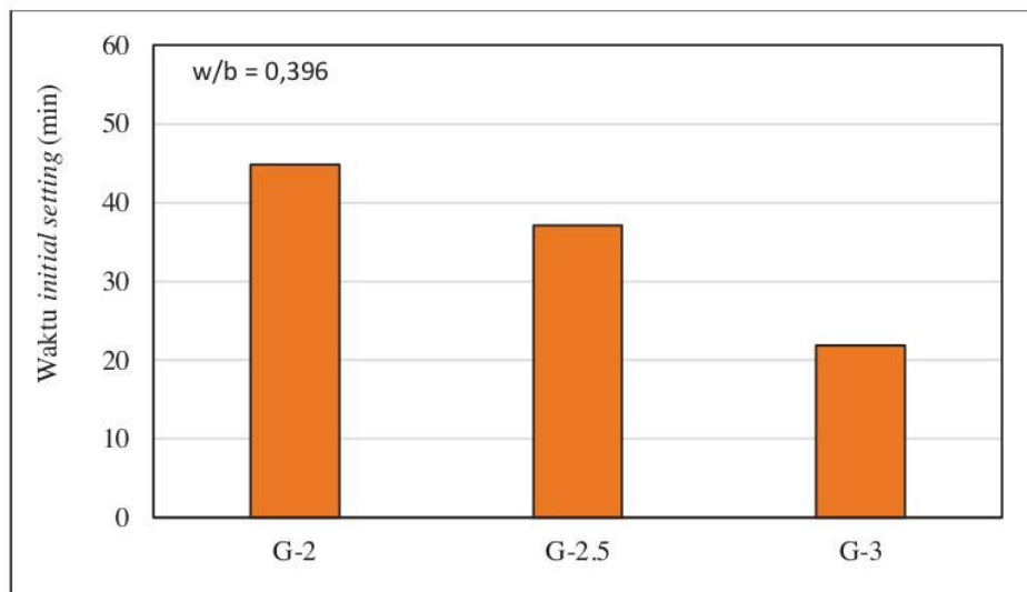
Gambar 8.1. Waktu initial setting mortar geopolimer.
