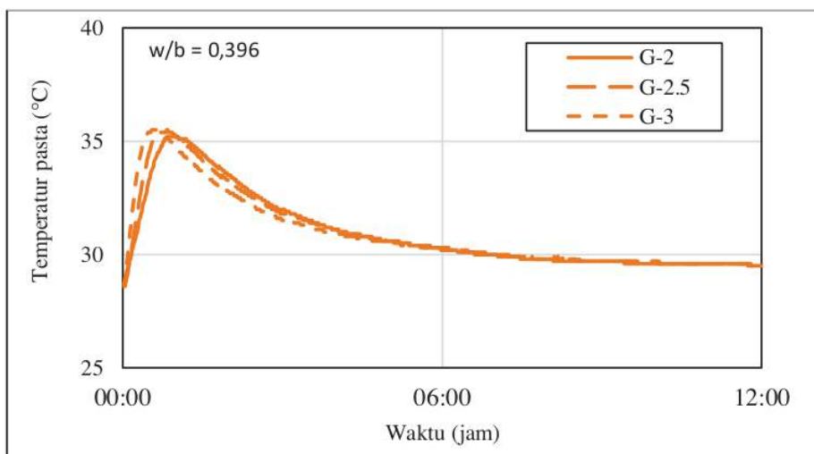
Gambar 8.2. Evolusi suhu pasta geopolimer.
