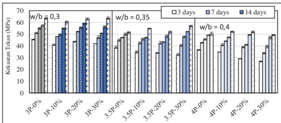
Gambar 5.4. Kekuatan tekan mortar pozzolan
