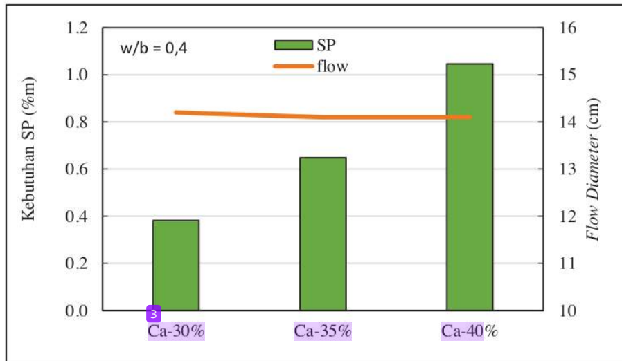
Gambar 7.1. Kebutuhan superplasticizer untuk mortar Fa-Ca
