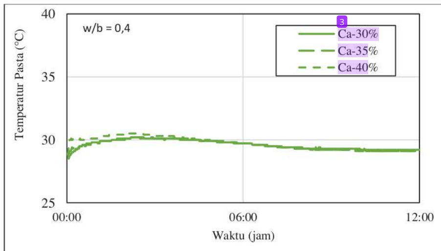
Gambar 7.3. Evolusi suhu campuran pasta Fa-Ca
