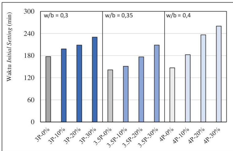
Gambar 5.2. Waktu pengikatan awal mortar pozzolan
