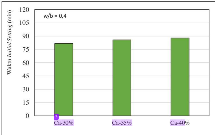
Gambar 7.2. Waktu pengikatan awal mortar Fa-Ca
