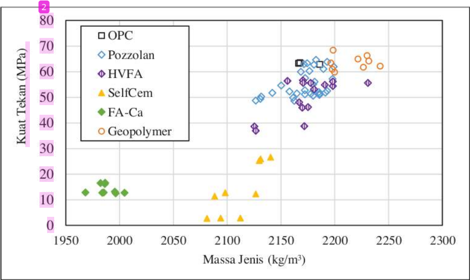
Gambar 8.4. Kuat tekan mortar yang dihasilkan sebagai fungsi dari massa jenisnya
