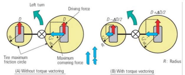
Gambar 2. Efek dari Torque Vectoring [4]
