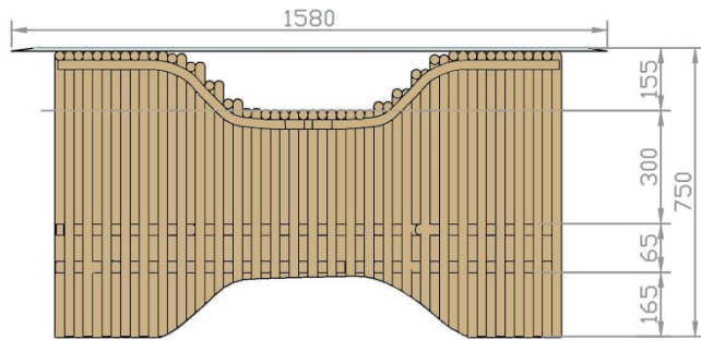
TAMPAK DEPAN
