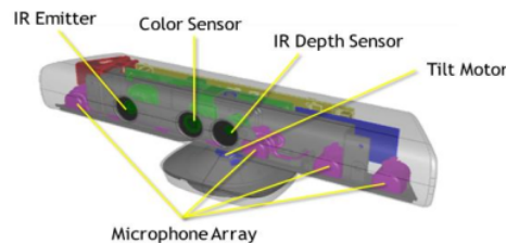
Gambar 1. Sensor-sensor pada Perangkat Kinect (Microsoft Library)
