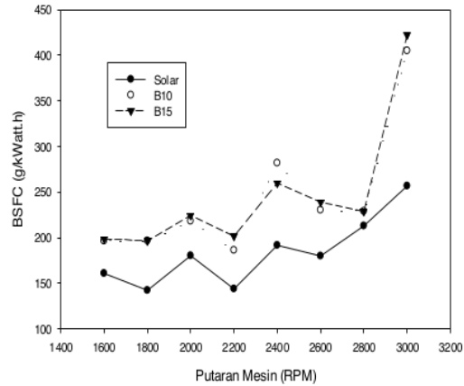
Gambar 7. Perbandingan BSFC terhadap putaran mesin
