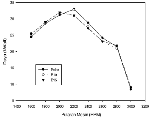
Gambar 5. Perbandingan daya terhadap putaran mesin
