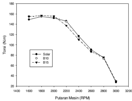
Gambar 6. Perbandingan torsi terhadap putaran mesin
