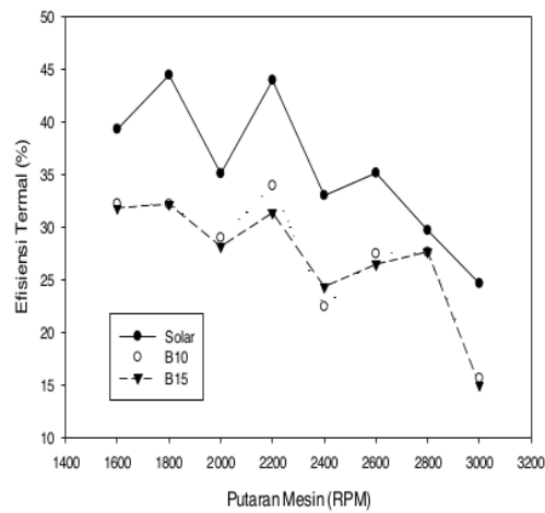
Gambar 8. Perbandingan brake thermal efficiency terhadap putaran mesin
