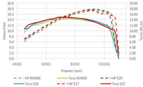
Gambar 3. Perbandingan Daya dan Torsi dengan menggunakan bahan bakar RON 90, E20 dan E27
