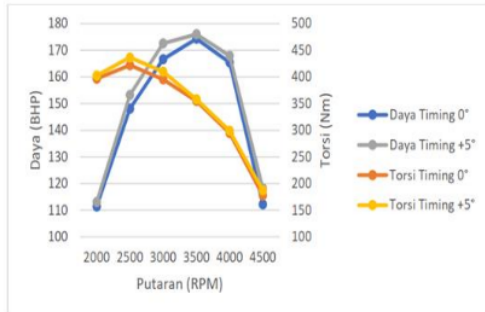
Gambar 3. Perbandingan Kinerja Mesin Diesel Injection Timing Bahan Bakar 0° dan +5°.
