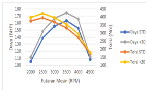
Gambar 2. Perbandingan Kinerja Mesin Diesel dengan Fuel Pressure Standard dan +20
