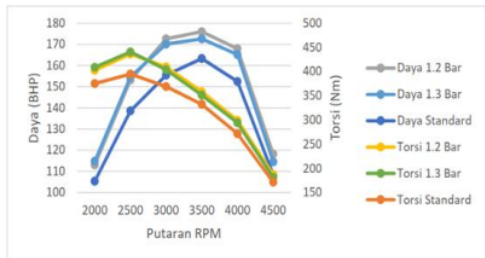
Gambar 4. Perbandingan Kinerja Mesin Diesel Tekanan Turbo Standard, 1.2 bar, dan 1.3 bar
