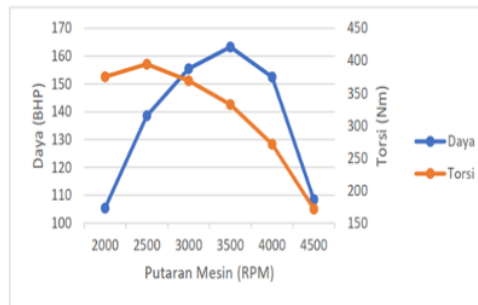
Gambar 1. Uji Dyno Mesin Standar
