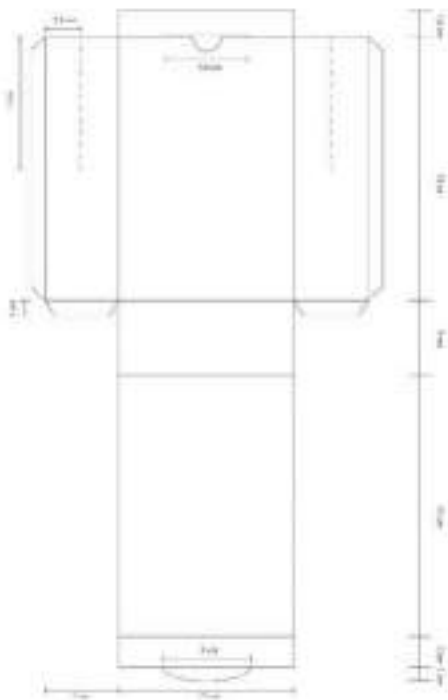
Gambar 34. Ukuran kemasan sekunder peach gum kering
