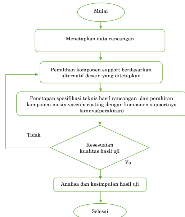
Gambar 4. Alur Perancangan dan Pembuatan serta Pengujian Mesin Vacuum Casting
