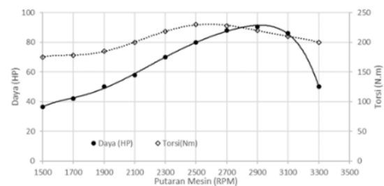
Gbr. 7 Kurva Daya dan Torsi Mesin Standar
