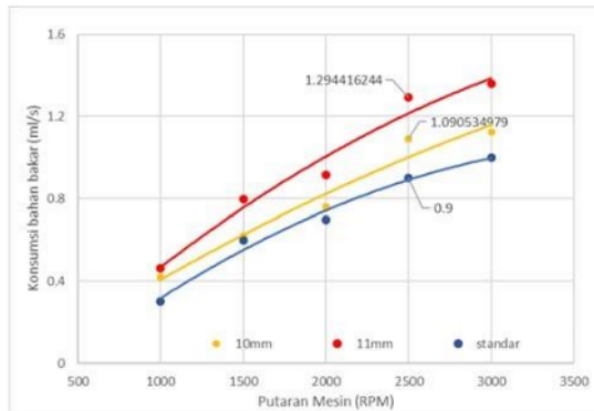
Gbr. 11 Kurva konsumsi bahan bakar
