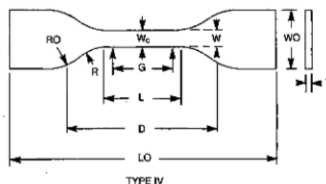
Gambar 4 Spesimen ASTM D638-4
