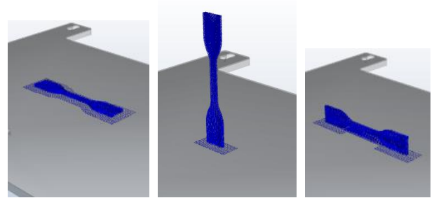
Gambar 12 Tampak Spesimen Setelah Build setting (a) Orientasi I, (b) Orientasi II, (c) Orientasi III
