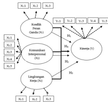
Gambar 1 Kerangka Konseptual
