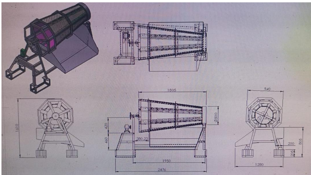
Gambar 1. Desain mesin pengayak sampah
