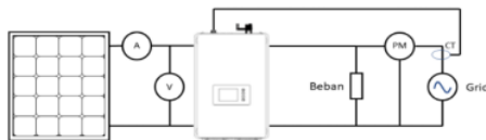
Gambar 6. Diagram titik pengukuran sistem
