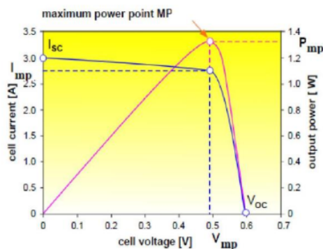
Gambar 1. Kurva karakteristik panel surya [2].
