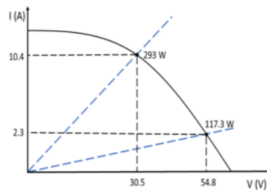
Gambar 7. Kurva I-V: Perubahan Titik Kerja Panel Surya.
