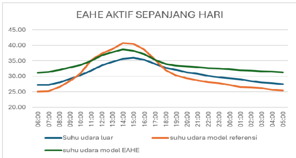
Gambar 2. Grafik pola temperatur udara 24 jam hasil eksperimen EAHE yang diaktifkan sepanjang hari. Sumber: Juniwati, 2021
