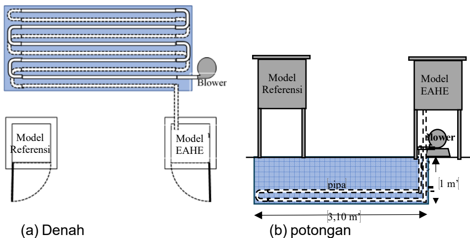
Gambar 4. Model Ruang Eksperimen (a) denah, (b) potongan
