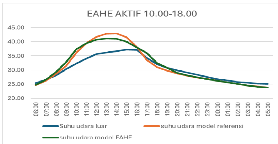
Gambar 5. Grafik pola temperatur udara 24 jam hasil eksperimen EAHE yang diaktifkan 10.00 – 18.00
