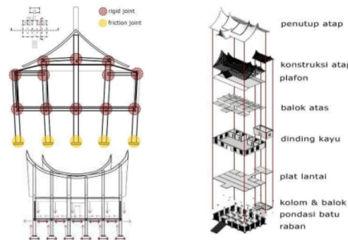
Gambar 5. Sistem penyaluran beban pada Bodi Caniago (sumber : analisis penulis, digambar berdasarkan data berbagai sumber [12,13])
