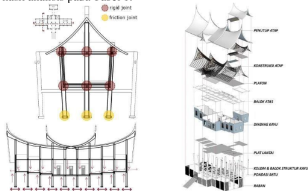
Gambar 4. Sistem penyaluran beban & Aksonometri Koto Piliang (sumber : analisis penulis, digambar berdasarkan data berbagai sumber [12,13])
