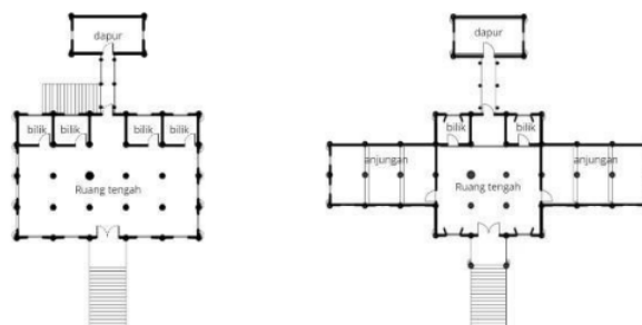
Gambar 6. Perbedaan bentuk denah Bodi Caniago dan Koto Piliang (sumber penulis, digambar ulang berdasarkan [10])
