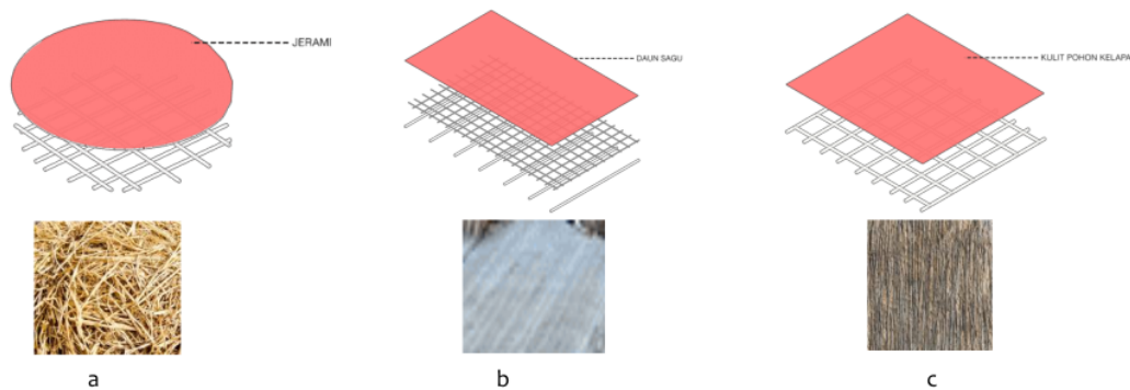
Gambar 8. Lantai dan material (a) rumah Honai, (b) rumah Jew, dan (c) rumah Yame Owaa Digambar ulang berdasarkan (a) Boissiere, 1999, (b) Fauziah, 2014 (c) Nawipa, 2004.
