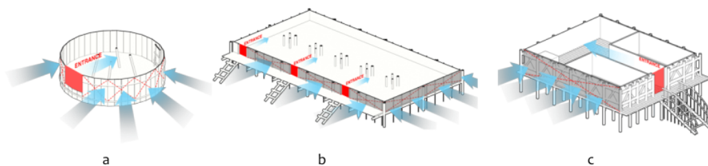
Gambar 7. Bukaannya pada (a) rumah Honai, (b) rumah Jew, dan (c) rumah Yame Owaa Digambar ulang berdasarkan (a) Boissiere, 1999, (b) Fauziah, 2014, (c) Mote, 2018.
