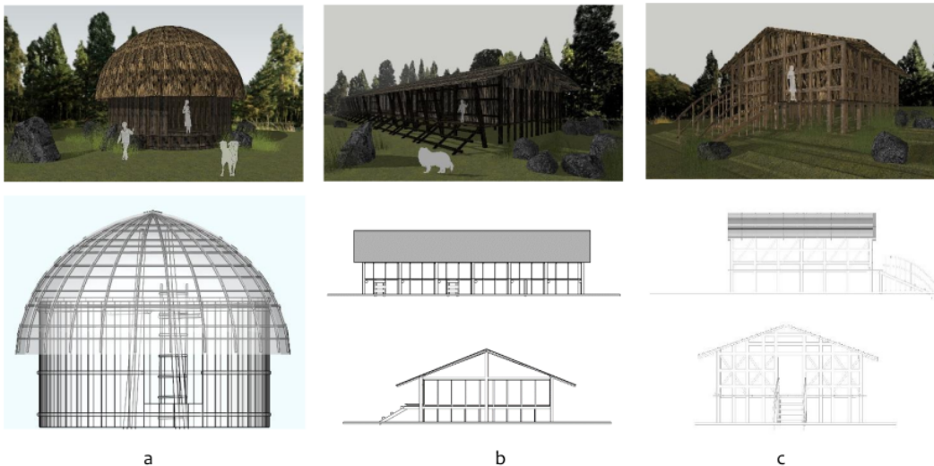
Gambar 4. Bentuk & denah (a) rumah Honai, (b) rumah Jew, dan (c) rumah Yame Owaa Digambar ulang berdasarkan (a) Agustinus, 1997., (b) Bitar, 2022., (c) Tekege, 2021.
