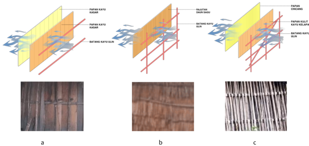
Gambar 9. Perbandingan dinding dan material (a) rumah Honai, (b) rumah Jew, dan (c) rumah Yame Owaa Digambar ulang berdasarkan (a) Boissiere, 1999., (b) Fauziah, 2014., (c) Nawwipa, 2004.
