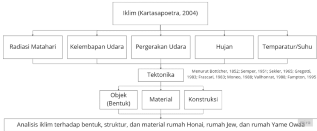
Gambar 3. Kerangka Teori
