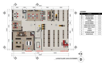
Gambar 12. Layout Glory Jaya Stationery (Sumber: Data penulis, 2024)
