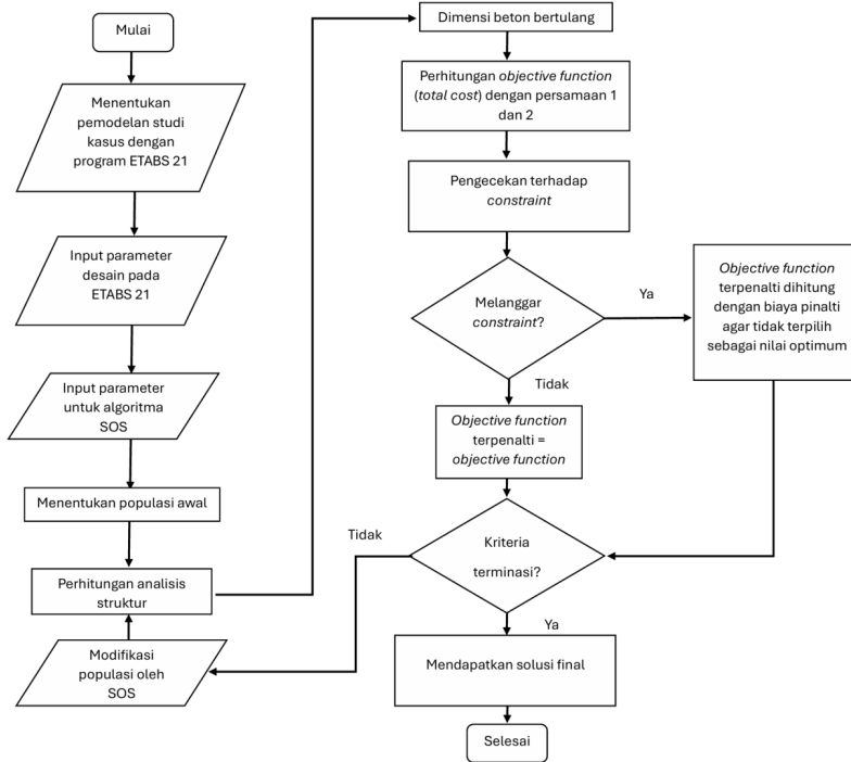
Gambar 1. Diagram alir proses optimasi menggunakan algoritma sybiotic organisms search (SOS)
