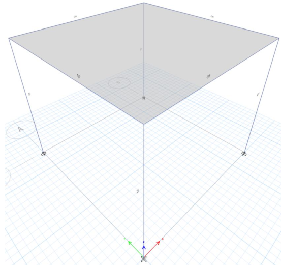
Gambar 2. Pemodelan struktur beton 3D pada ETABS
