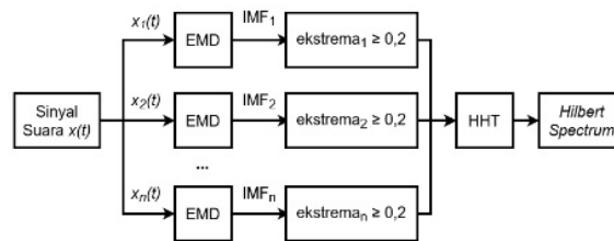
Gbr. 4 Diagram alir spektrum Hilbert dengan HHT.
