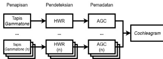
Gbr. 2 Model koklea sebagaimana diadaptasi dari Lyon [20].
