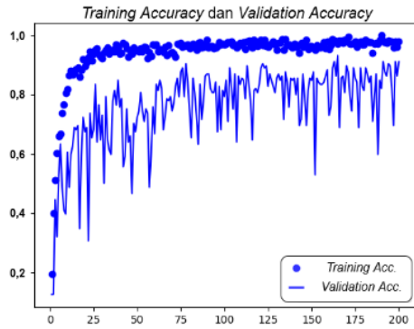
Gbr. 6 Grafik rerata akurasi dengan CNN (komposisi data 80:20).
