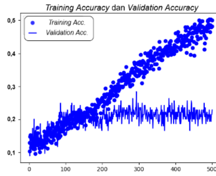
Gbr. 8 Grafik rerata akurasi dengan LSTM (komposisi data 80:20).
