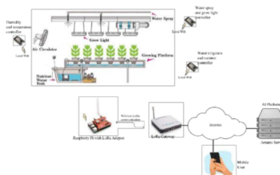
Gambar 3. Disain sistem IoT untuk mendukung smart urban farming pada kebun hidroponik
