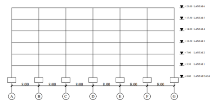
Gambar 6. Portal Tipikal dari Struktur yang Ditinjau
