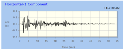
Gambar 8. Gempa Imperial Valley (El Centro 1940) Horizontal 1
