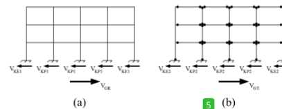
Gambar 2. Pemodelan Struktur M-PCD: (a) Model Ke-1; (b) Model Ke-2
