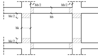
Gambar 1. Dimensi Bagian yang Direduksi Kekakuan Lenturnya
