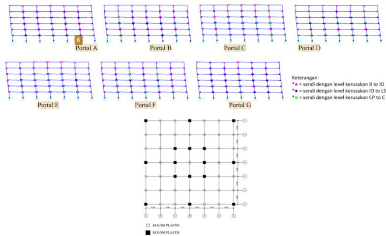
Gambar 13. Mekanisme Kerusakan Bangunan B pada Level Gempa MCER
