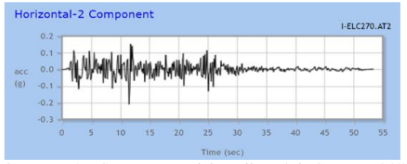
Gambar 9. Gempa Imperial Valley (El Centro 1940) Horizontal 2
