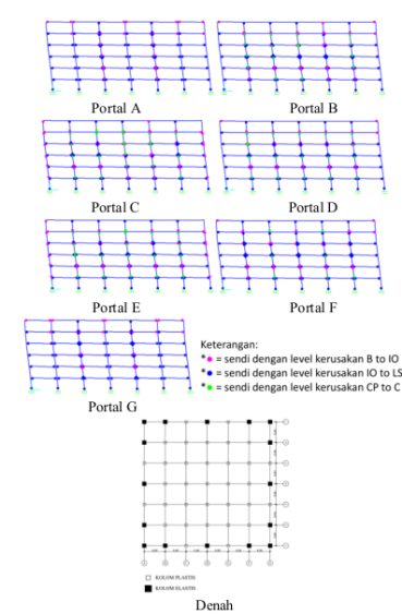
Gambar 11. Mekanisme Kerusakan Bangunan A pada Level Gempa MCER
