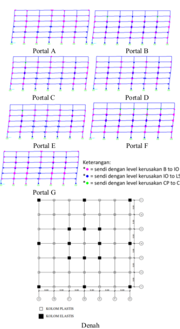
Gambar 12. Mekanisme Kerusakan Bangunan B pada Level Gempa EDRS
