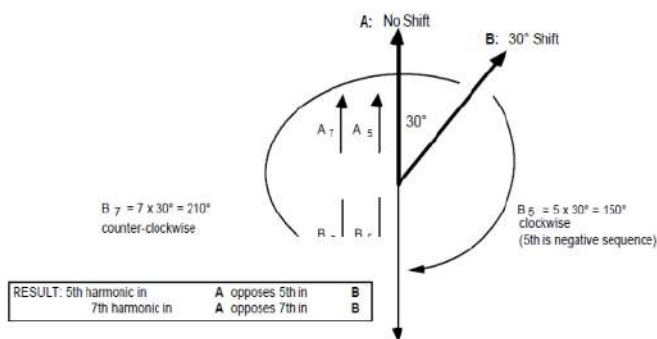
Gambar 3. Pergeseran fasa 30^\circ Menghilangkan Harmonisa Arus ke 5 dan ke 7
