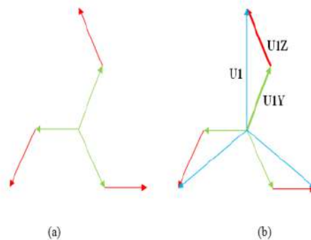
Gambar 1. (a) Rangkaian Zig-Zag (b) Resultan 0^0 Pada Rangkaian Zig-Zag
