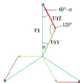
Gambar 2. Rangkaian Zig-Zag Dengan Pergeseran Berbagai Sudut Fasa
