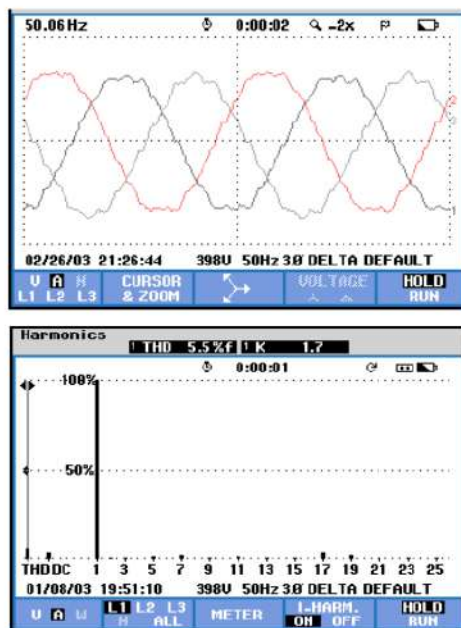
Gambar 7. Gelombang Arus dan Spektrum Harmonisa setelah Menggunakan Transformer Penggeser Fasa
