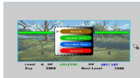
Gambar 12. Duel Mode
