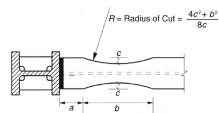
Gambar 4.4 Spesifikasi RBS yang Digunakan
