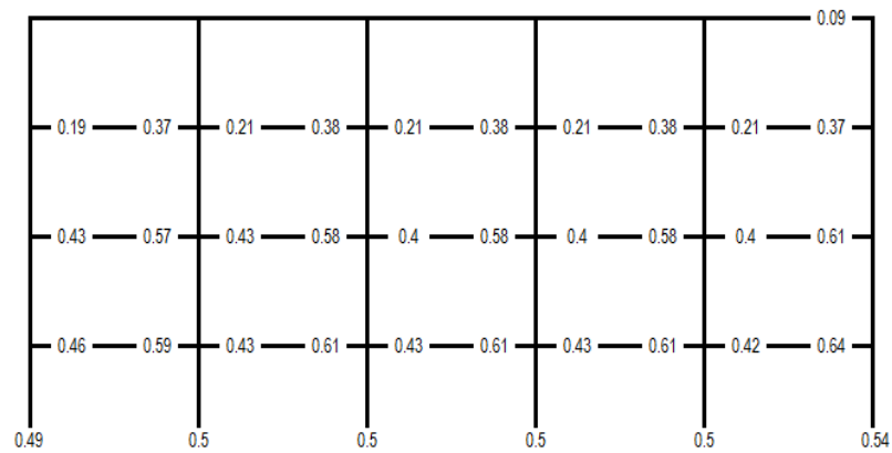
Gambar 5.15 Lokasi Terjadinya Sendi Plastis dari Hasil Analisis Time History untuk Bangunan 4-lantai pada Portal Interior 1000 Tahun
