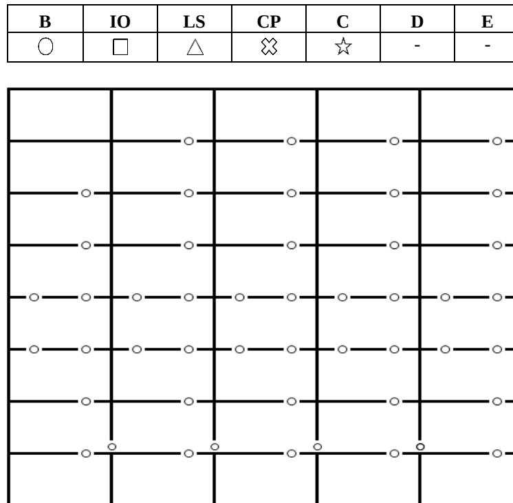
Gambar 5.16 Lokasi Terjadinya Sendi Plastis dari Hasil Analisis Pushover untuk Bangunan 8-lantai pada Portal Eksterior 100 Tahun
