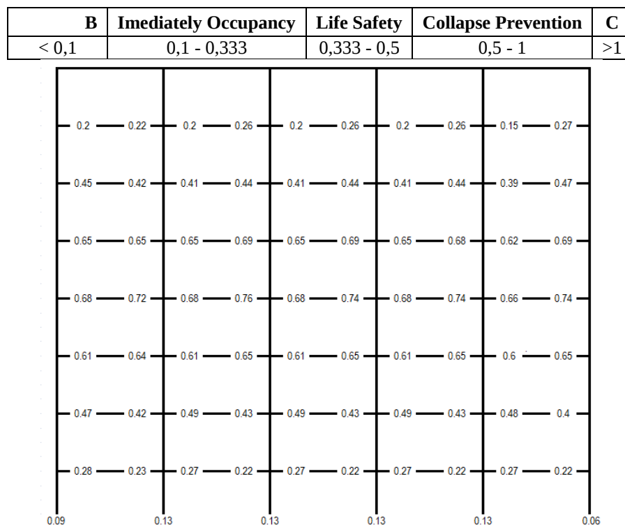
Gambar 5.27 Lokasi Terjadinya Sendi Plastis dari Hasil Analisis Time History untuk Bangunan 8-lantai pada Portal Interior 1000 Tahun
