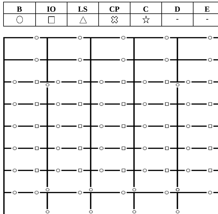
Gambar 5.26 Lokasi Terjadinya Sendi Plastis dari Hasil Analisis Pushover untuk Bangunan 8-lantai pada Portal Interior 1000 Tahun
