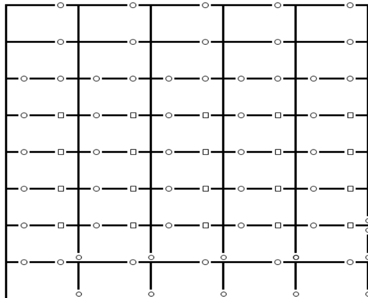
Gambar 5.22 Lokasi Terjadinya Sendi Plastis dari Hasil Analisis Pushover untuk Bangunan 8-lantai pada Portal Interior 500 Tahun
