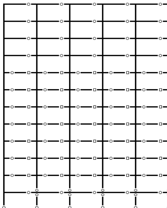
Gambar 5.31 Lokasi Terjadinya Sendi Plastis dari Hasil Analisis Pushover untuk Bangunan 12-lantai pada Portal Interior 500 Tahun
