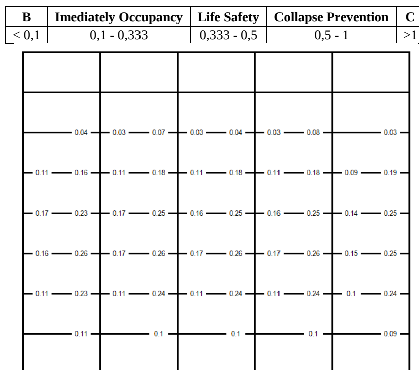
Gambar 5.17 Lokasi Terjadinya Sendi Plastis dari Hasil Analisis Time History untuk Bangunan 8-lantai pada Portal Eksterior 100 Tahun
