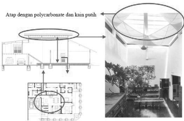
Gambar 11. Analisis Pembentuk Interior pada Renon House.
