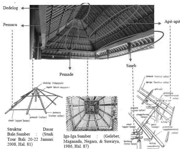
Gambar 2. Analisis plafon (atap ekspose) pada Balkon Utama di Lantai 4 The Long House Villa.
