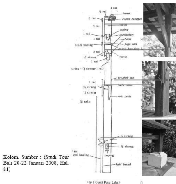
Gambar 6. Analisis Model Tiang (saka) di area Museum Pasifika.
